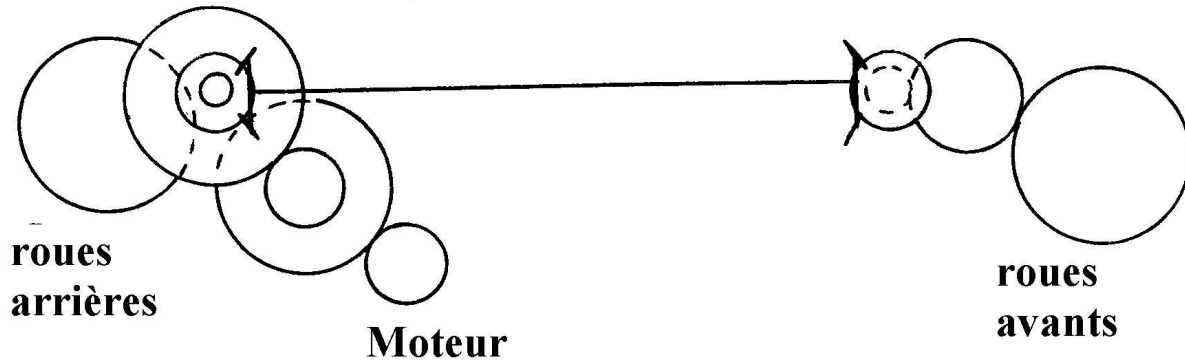
TRANSMISSION TAMIYA Boîte courte (sans les liaisons pivot)
